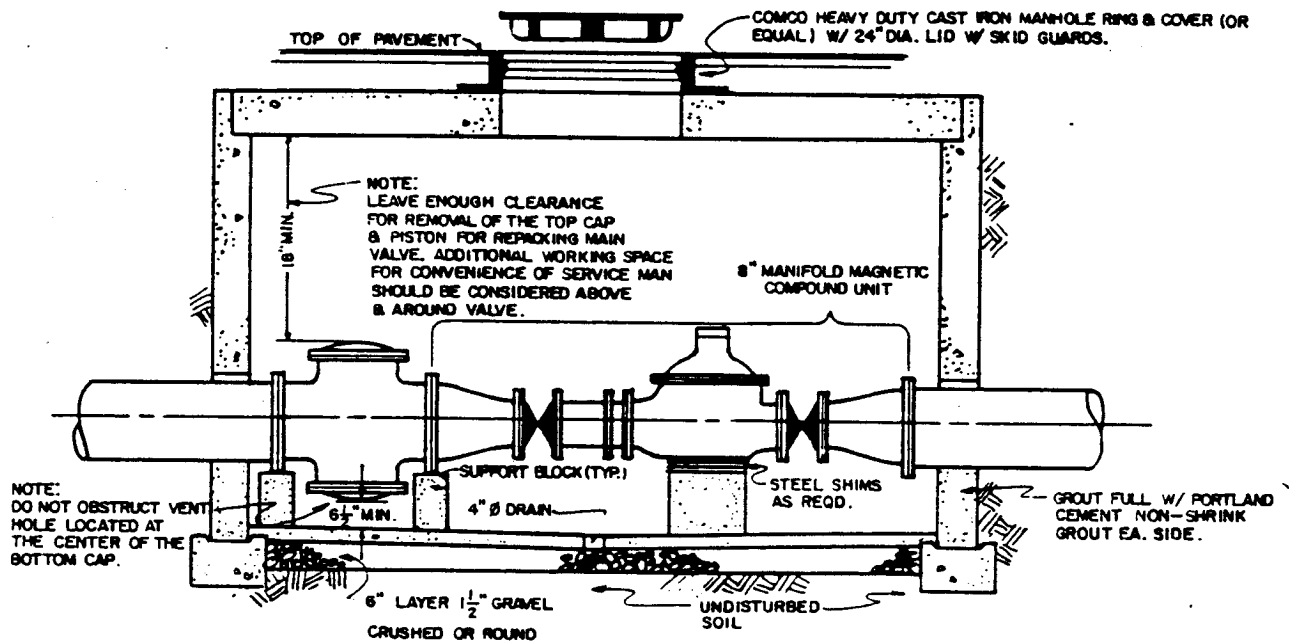
SECTION A-A
